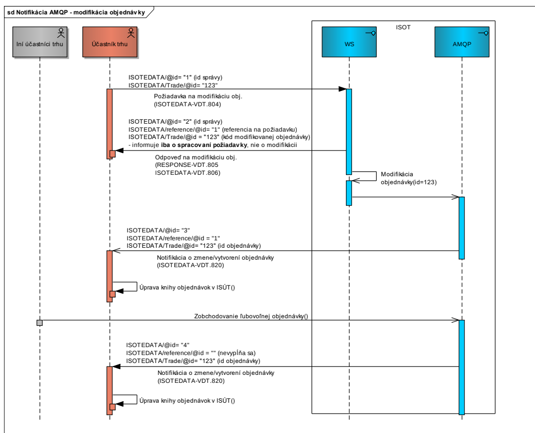
Obrázok 32 Schéma následnosti posílaných správ – modifikácia objednávky (AMQP notifikácia)
